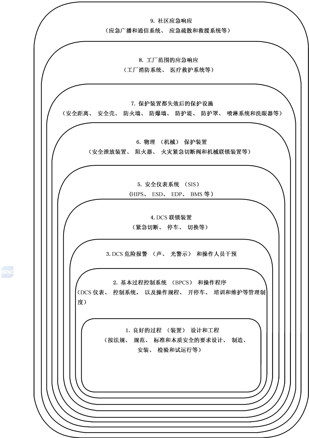
图 A.1 典型的安全保护层图
